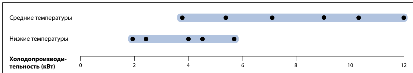
Компрессорно-конденсаторные агрегаты для установки вне помещений Copeland EazyCool ZX со спиральными компрессорами
