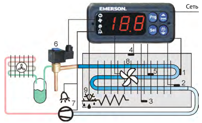
Контроллер торгового оборудования EC2-31x / -39x (EX2, темп./темп.)
