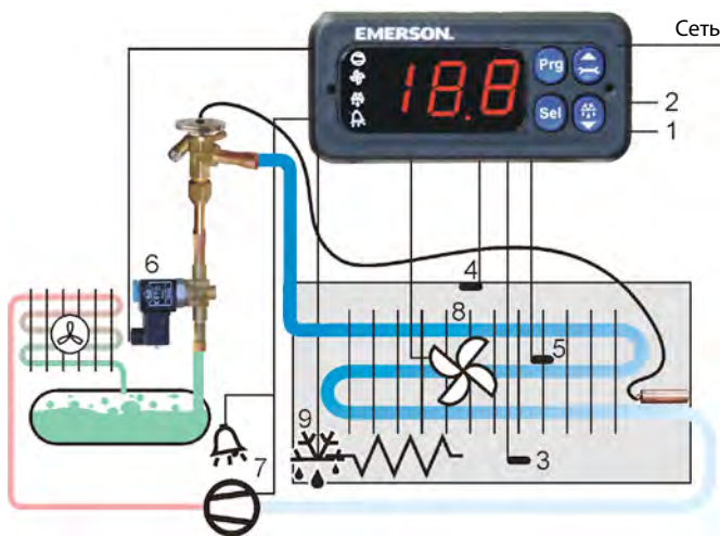
Контроллер торгового оборудования (ТРВ) EC2-21x/-29x
