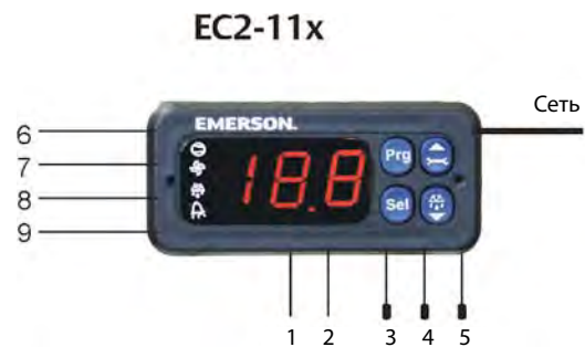
Универсальный контроллер ввода-вывода EC2-11x
