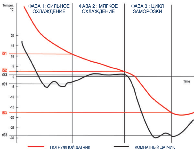
На рисунке показан типичный цикл заморозки
